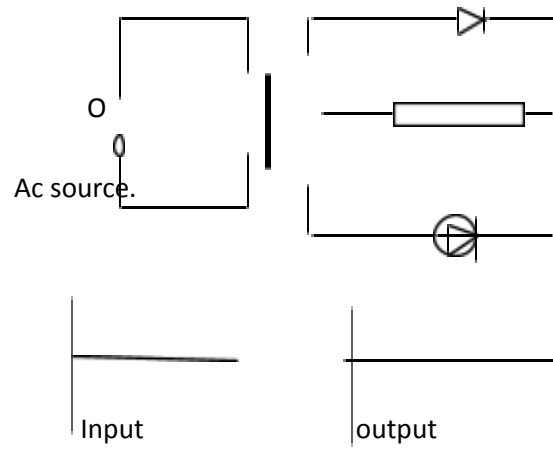
CENTRE-TAP FULL WAVE rectifier
