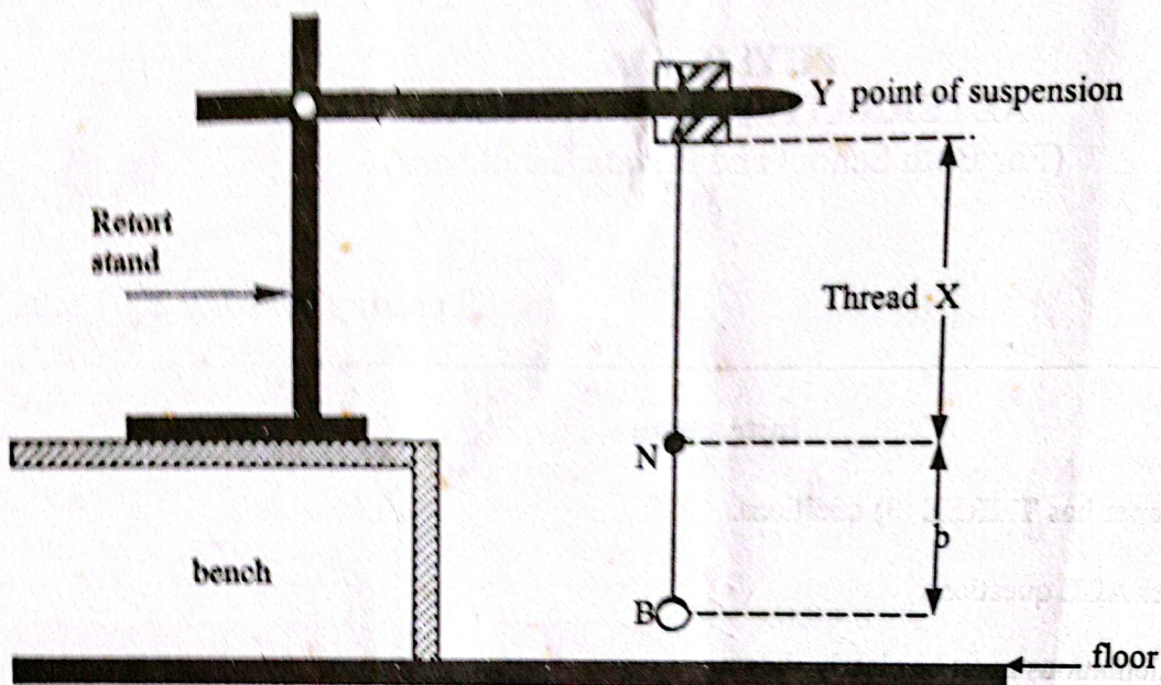
Fig 1. Simple Pendulum.
